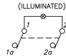
CIRCUIT: DPST
