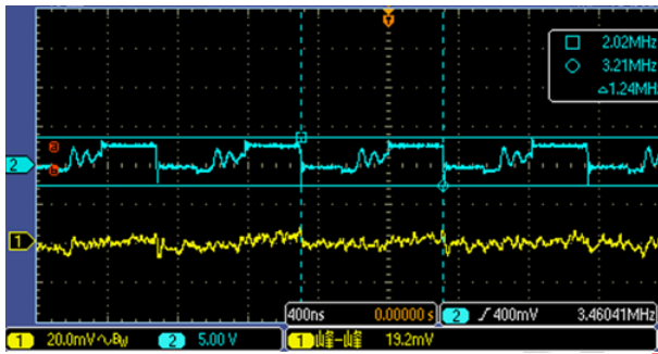
VIN = 2.7V, ILOAD = 0.1A Waveform
