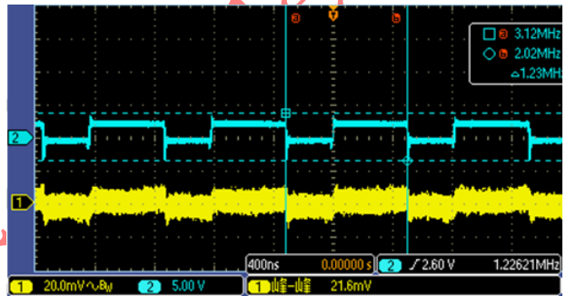
VIN = 2.7V, ILOAD = 1A Waveform
