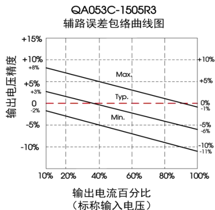
图 4 (辅路误差包络曲线)
