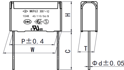
W \pm 0.4, H \pm 0.4, T \pm 0.4 圆弧底(Arc-bottom)
