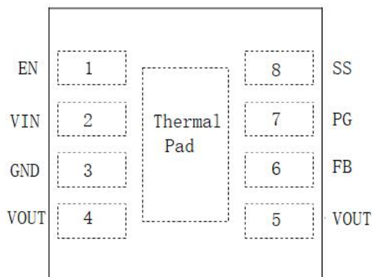
顶视图 (透视)
