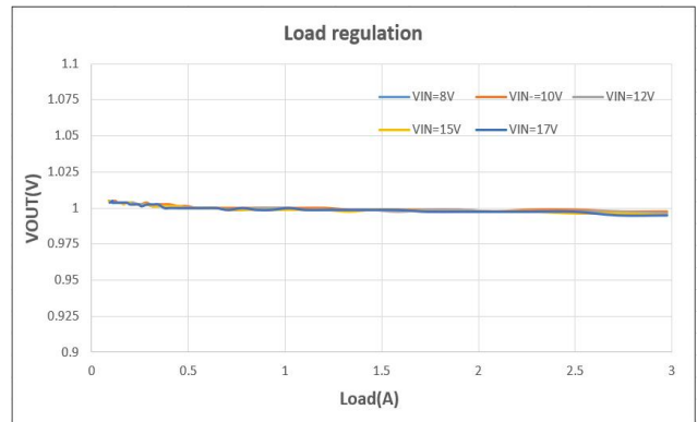
负载调整率 ( V_{OUT} = 1.0V )
