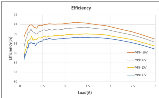
输出电流 vs 效率 ( V_{OUT} = 5.05V )
