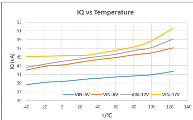
静态电流
