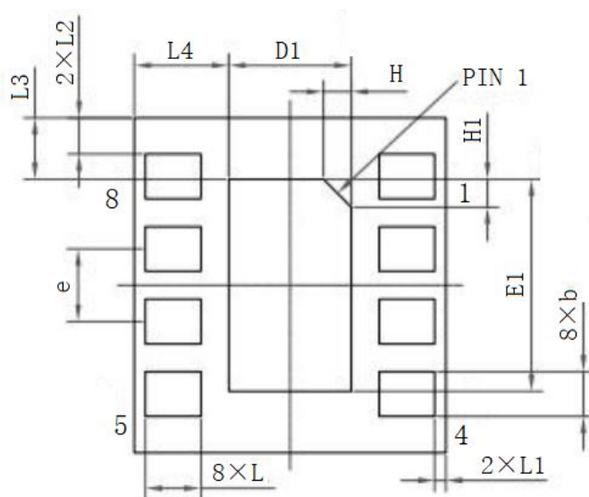
底视图
