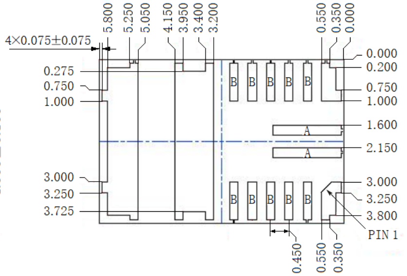
底视图
