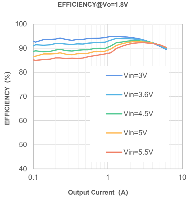
输出电流 vs 效率 (VOUT=1.8V)
