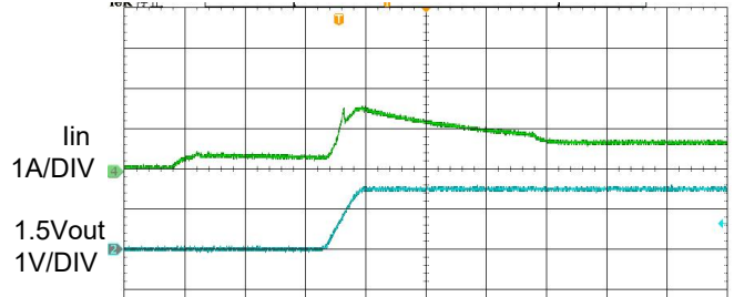
输出启动-4A负载
