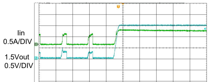
输出短路移除-4A负载 (瞬态, 打嗝模式)
