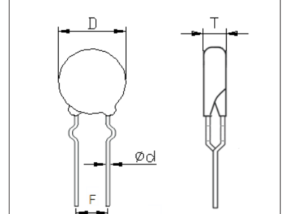
圖9: 外彎+Y脚 (D) Fig-9: Outside Kink & Y Type (D)
