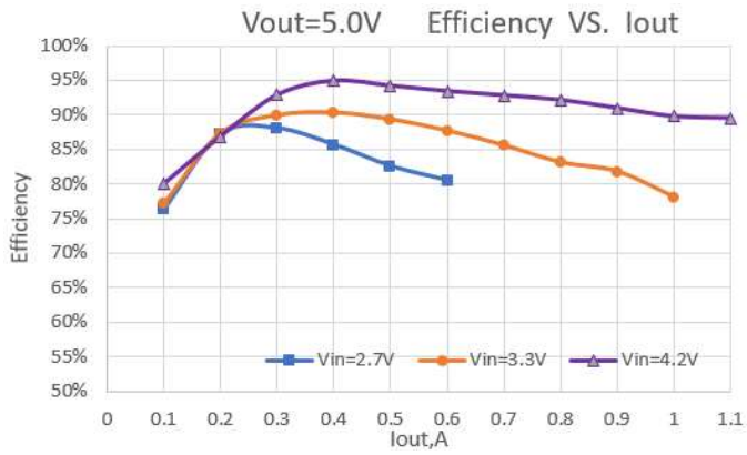
效率
