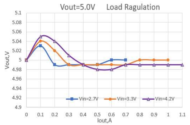
负载调整率
