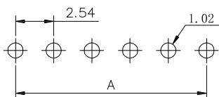
PCB参考图
