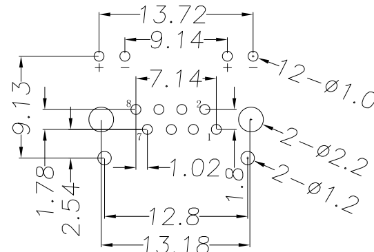
PCB参考图
