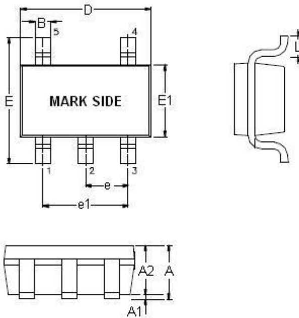
TSOT-23-5 Package (Unit: mm)
