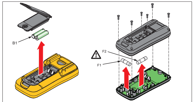
图 5. 更换电池和保险丝
