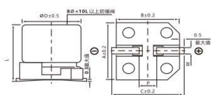
∅D=4~10 适用
