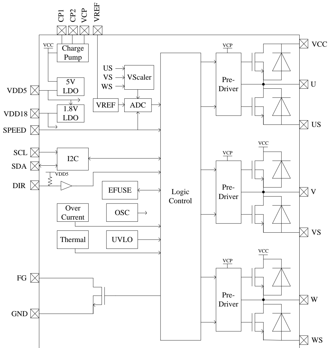
图 1-2 FT8213 功能框图
