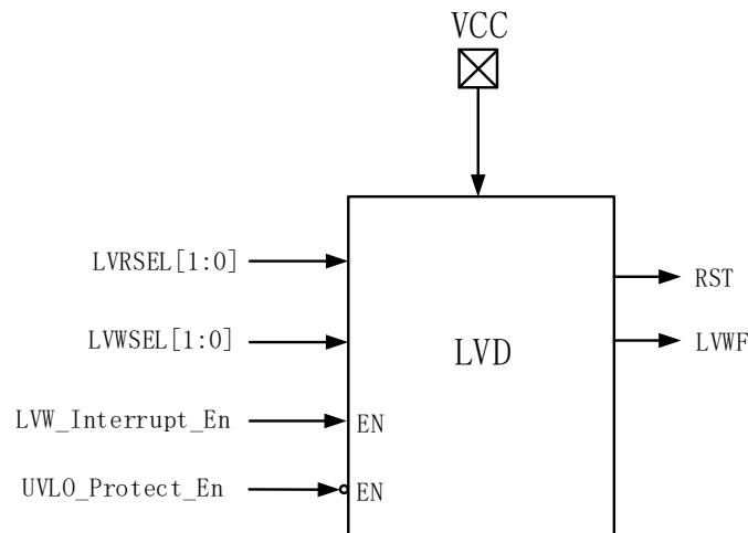
图 21-1 低电压检测模块
