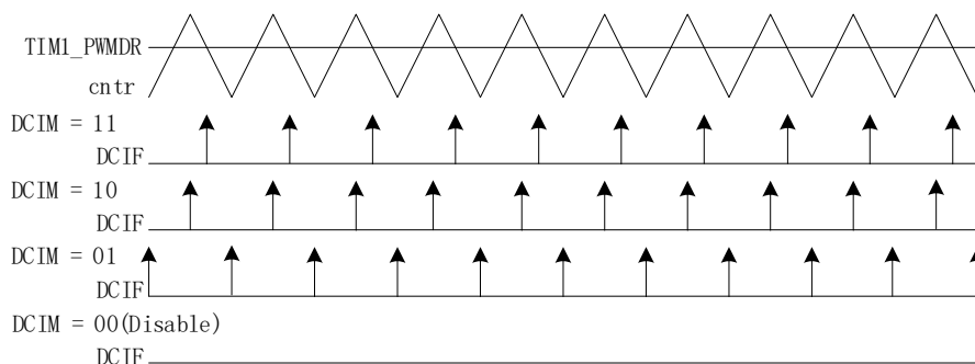
图 15-8 Driver 比较匹配中断
