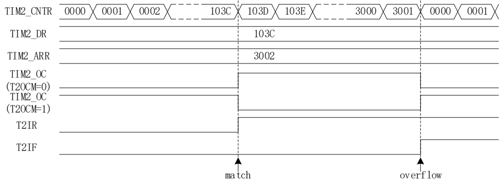
图 11-2 输出模式输出波形
