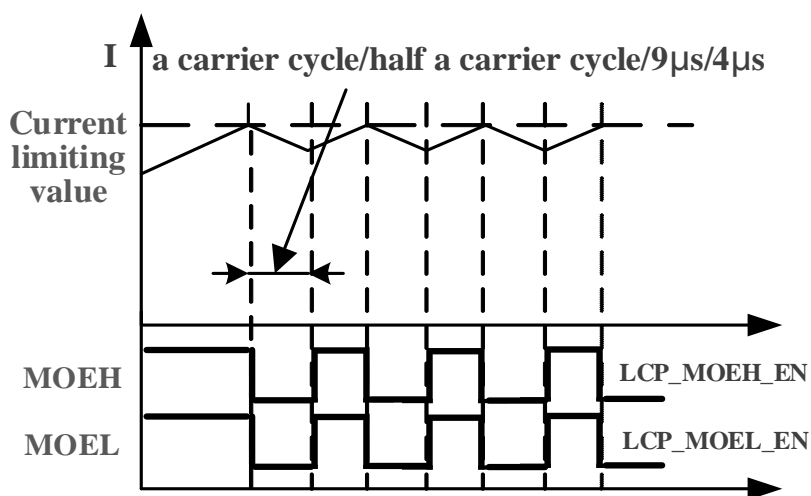
图 20-4 逐波限流
