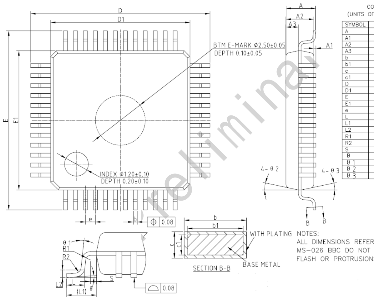
图 4-1 LQFP48_7X7 封装尺寸图
