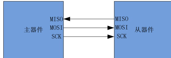
图 7-2 3 线单主方式和 3 线单从方式连接图
