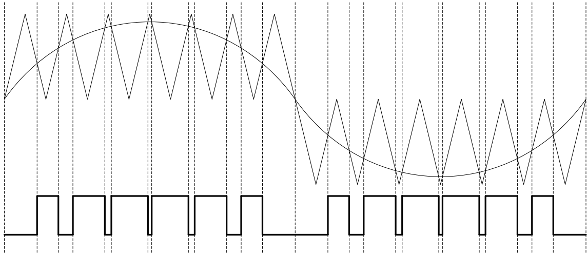
图 12-6 单极性 SPWM
