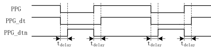
图 15-14 带死区插入的互补输出
