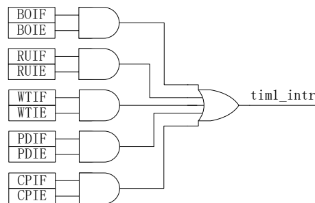
图 15-17TIMER1 中断源
