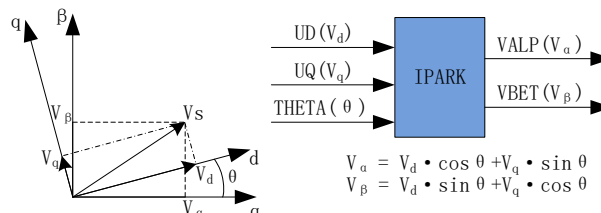
图 13-2 PARK 逆变换
