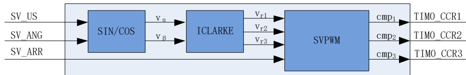
图 12-1 SVPWM 原理框图
