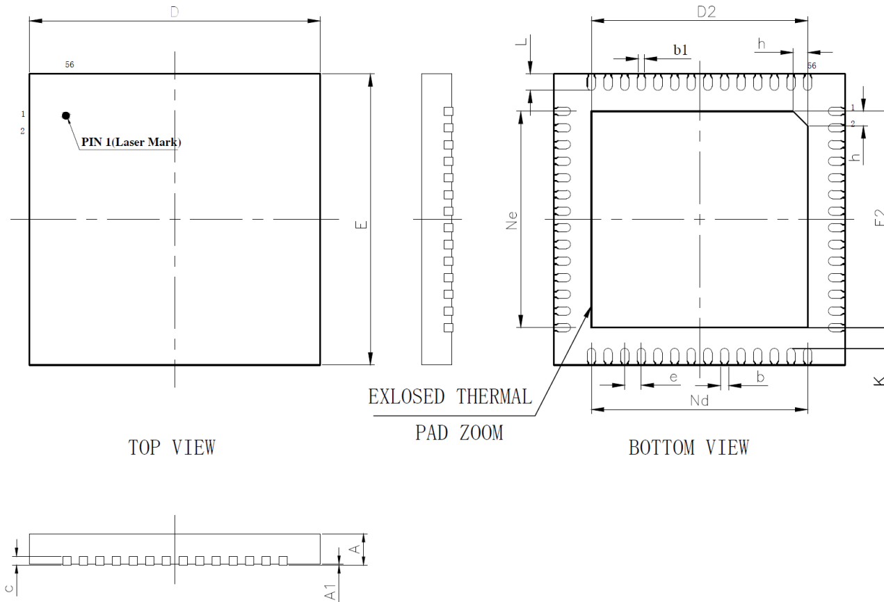
图 34-3 QFN56_7X7 封装尺寸图
