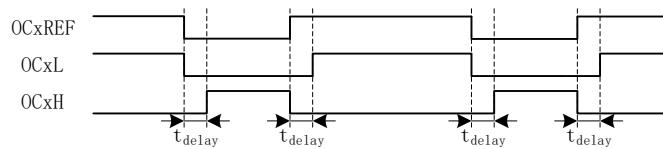
图 13-20 带死区插入的互补输出
