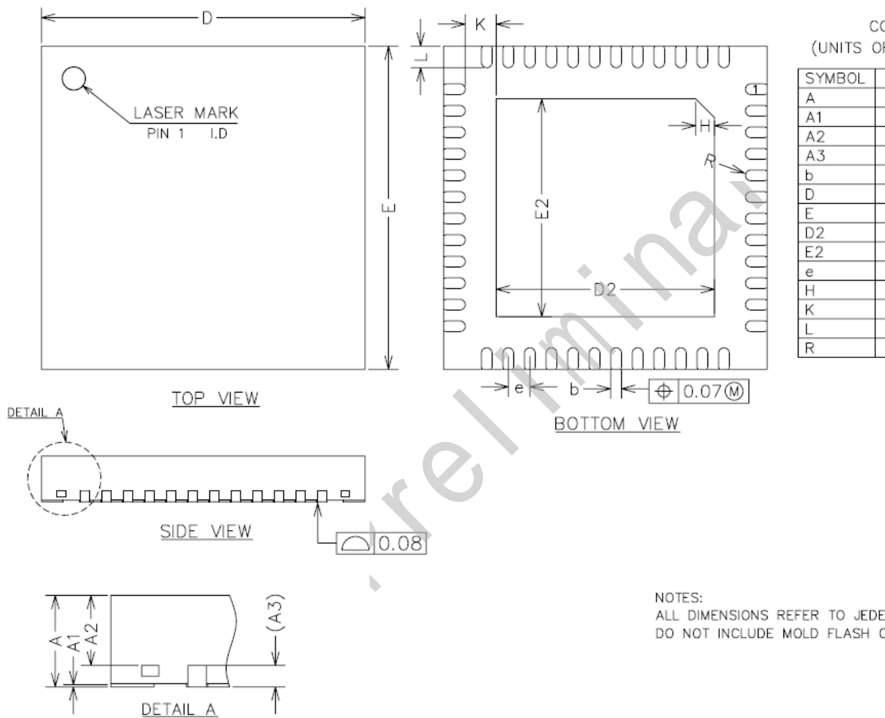
图 4-2 QFN48_6X6 封装尺寸图
