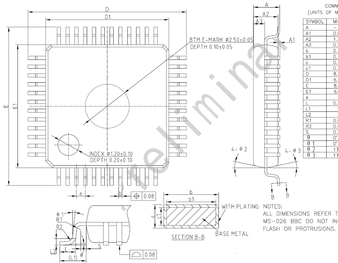
图 4-1 LQFP48_7X7 封装尺寸图
