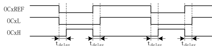
图 18-6 带死区插入的互补输出
