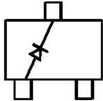
SOT-23 封装内部結構
