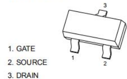
SOT-23 -3L
