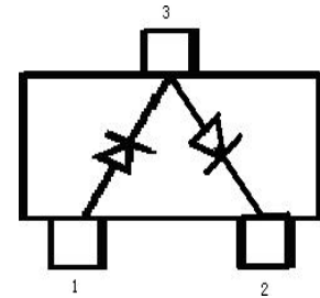
SOT-23 内部结构
