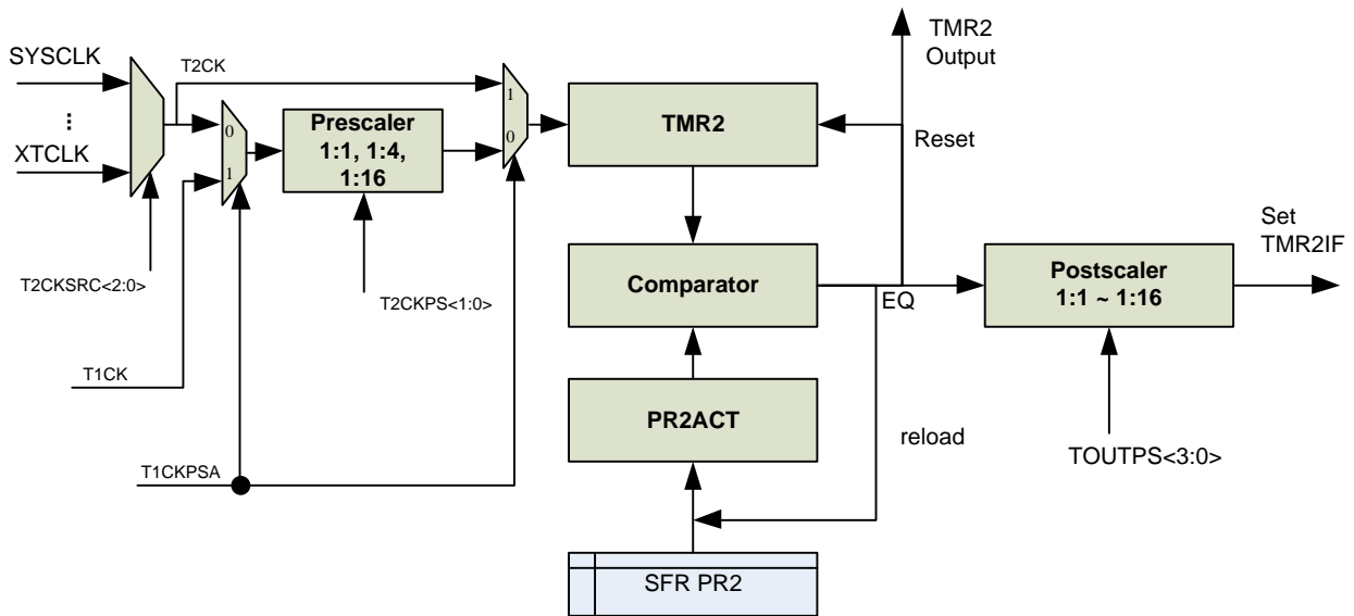
图 12.1 定时器 2 框图
