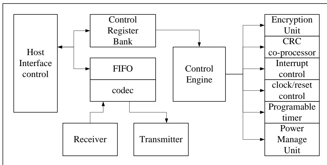
图 1-1 FM17522E 结构框图
