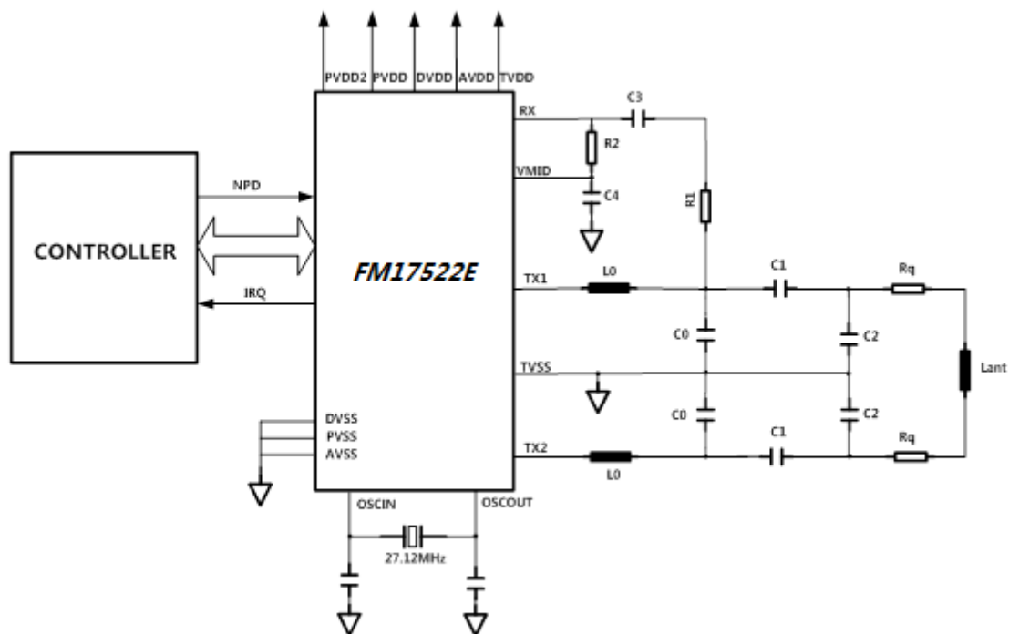
图 16-1 典型应用图
