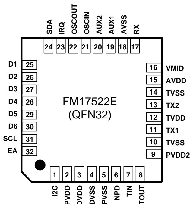
图 1-2 FM17522E QFN32 封装引脚图 (TOP VIEW)
