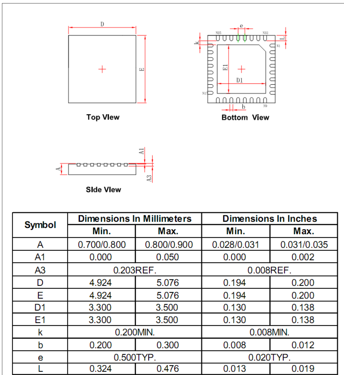
图 19-1 FM17522E QFN32 封装尺寸图
