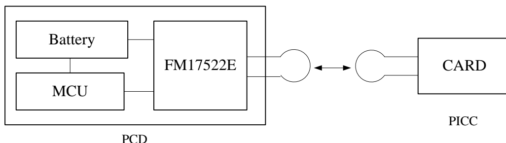
图 2-1 FM17522E 应用框图
