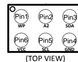
Thin 6-ball WLCSP (CTB)
