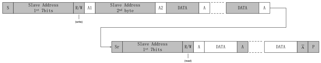
图 12-18 I2C 软件发送数据流程图
