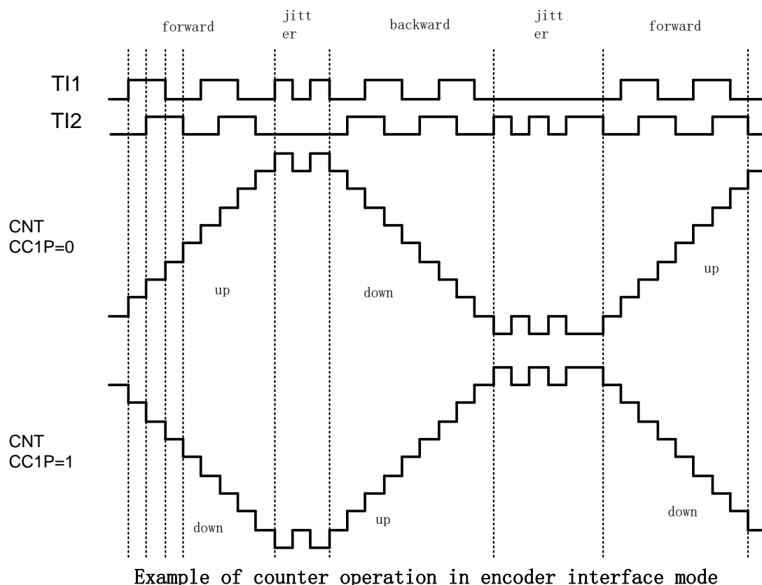
图 20-32 编码器模式下的计数器操作实例
