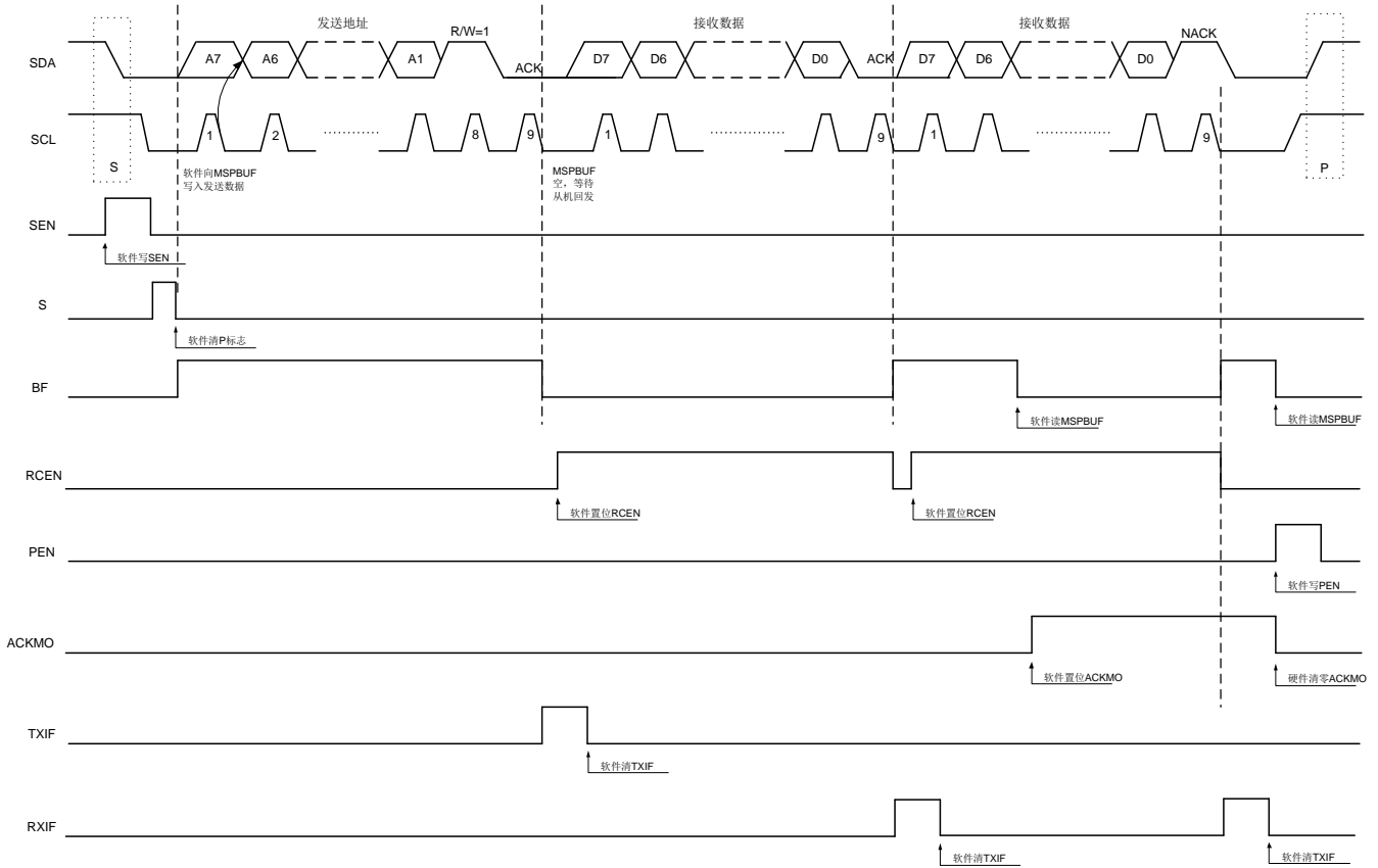
图 12-12 I2C 从 7 位地址从机读取数据流程图
