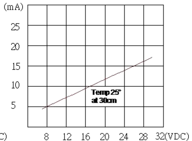
mA-V
