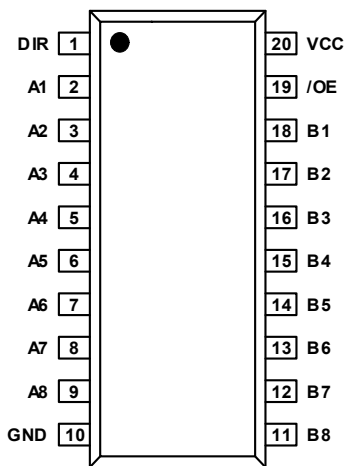
SOP-20/TSSOP-20
