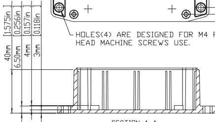
SECTION A-A SCALE 2 : 3
