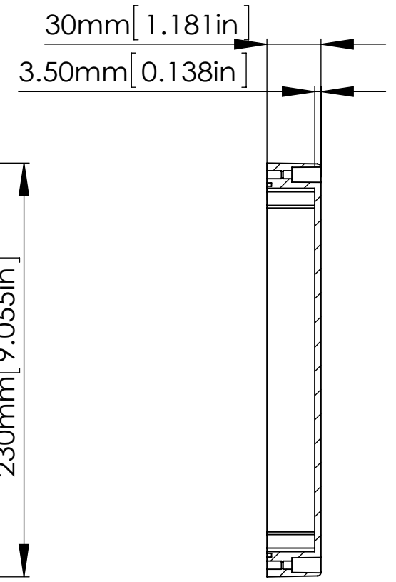
SECTION B-B SCALE 1 : 3
