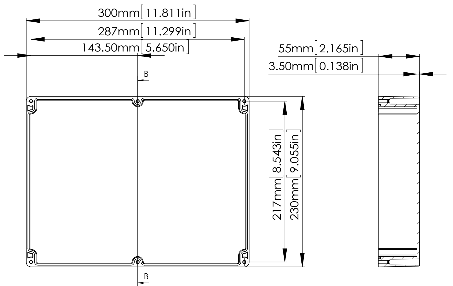
SECTION B-B SCALE 1 : 3
