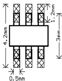
SOT-23-6/TSOT-23-6
