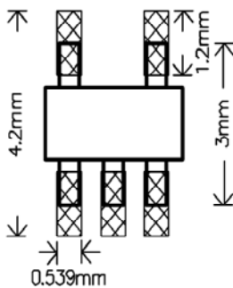
SOT-23-5/TSOT-23-5
