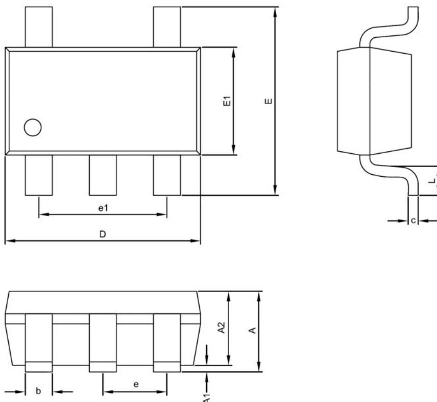
SOT-23-5 Package
