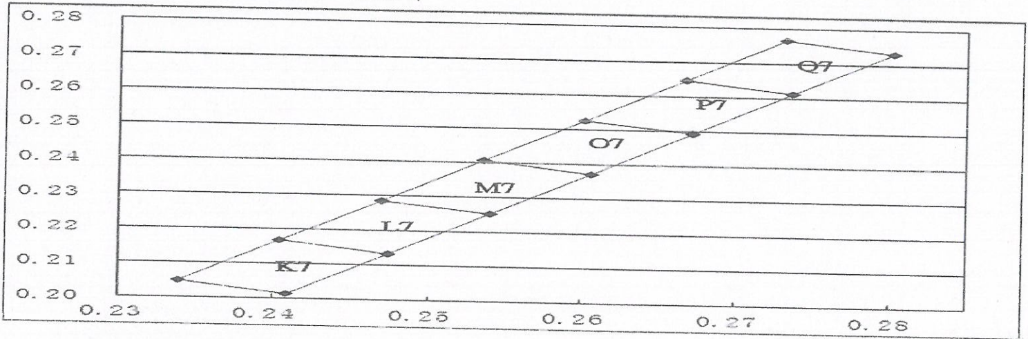
色度坐标分档 Color Bin Code (If=20mA)
