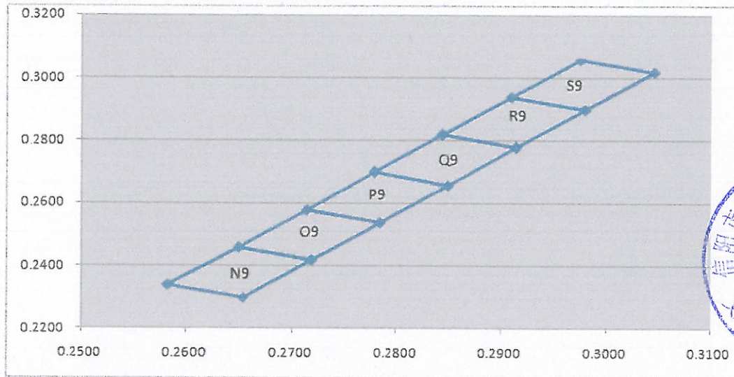
色度坐标分档 Color Bin Code (I f =20mA)
