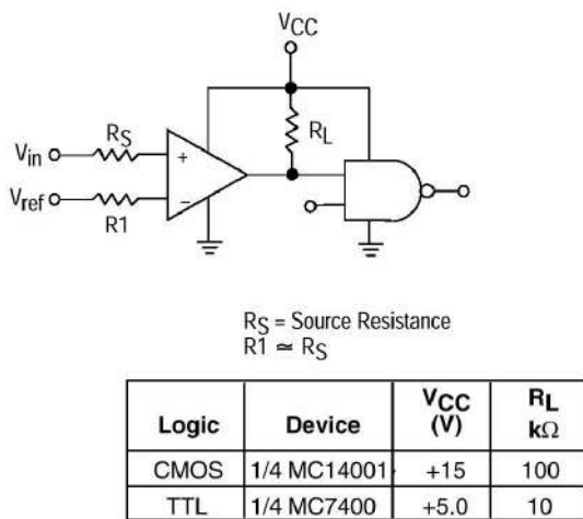
逻辑驱动器
