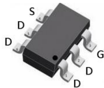
SOT-23-6
