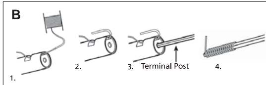
▲ Wrapping Wire
