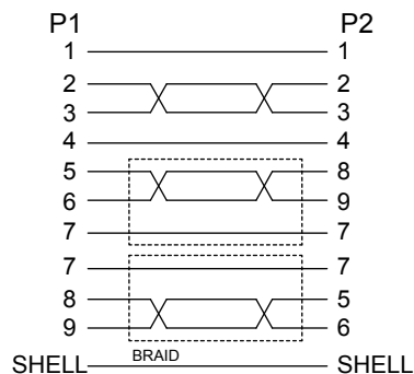
Anschlussdiagramm / Wiring diagram
