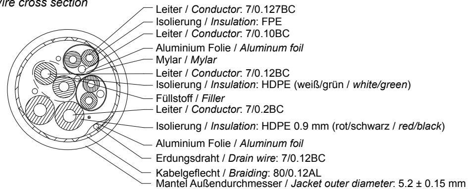
Aderquerschnitt / Wire cross section
