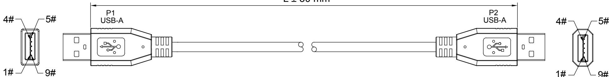
Anschlussdiagramm / Wiring diagram
