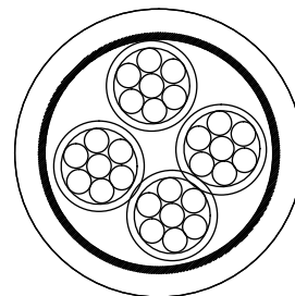
Aderquerschnitt / Wire cross section
