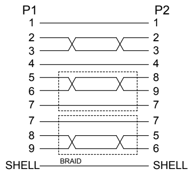
Anschlussdiagramm / Wiring diagram
