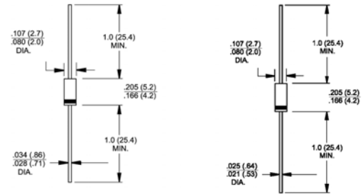
DO-204AL (DO-41)
