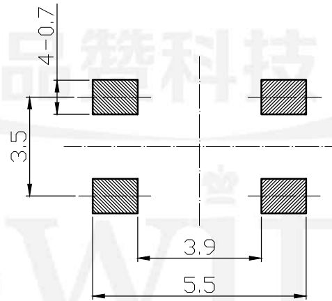
PCB. 焊接尺寸图
