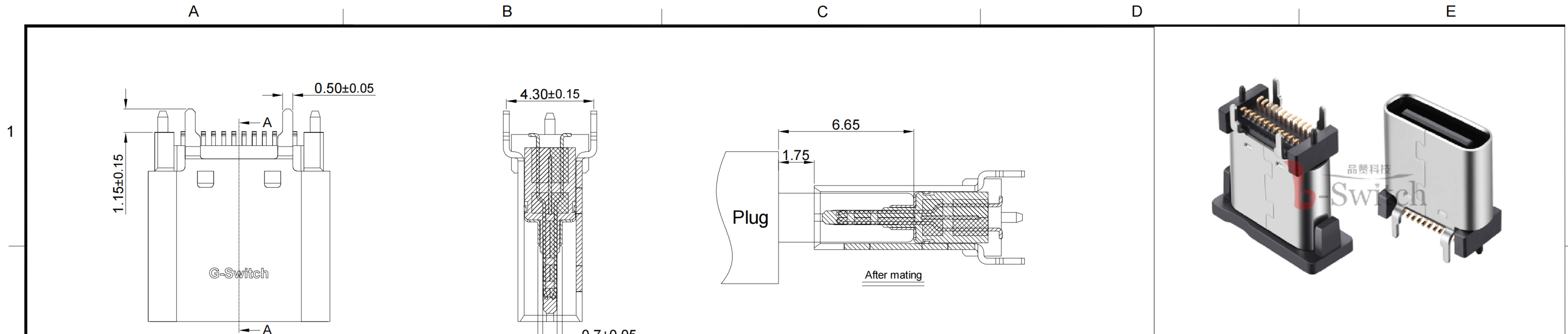
SECTION A-A
