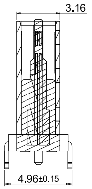
截面 1-1
