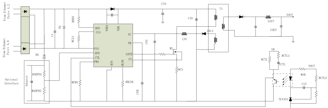
图17.反激变换器
