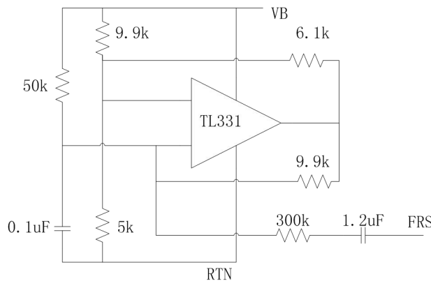
图24. 频率抖动
