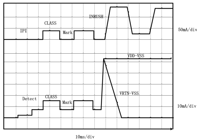
图13. Startup
