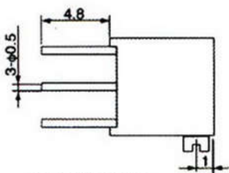
3266X型 (侧调)
