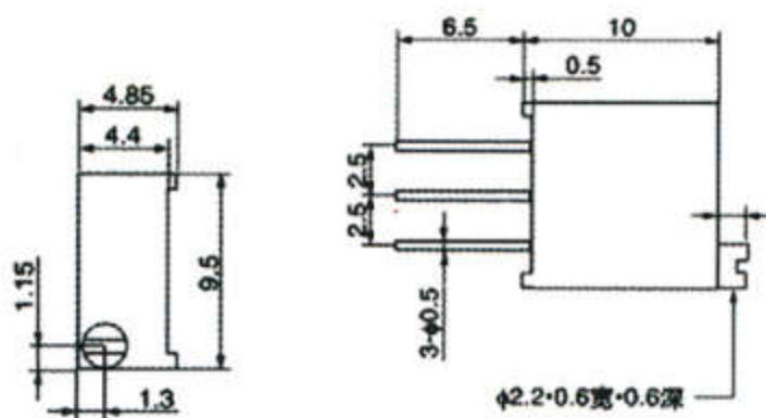
共有尺寸图
