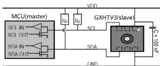
图 6 GXHTV3 的典型应用电路，包括上拉电阻和去耦电容 为了机械应力考虑，中心焊盘必须被焊接到地。
