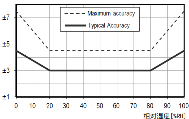
图 2 典型湿度误差和最大湿度误差 (@25° C)
